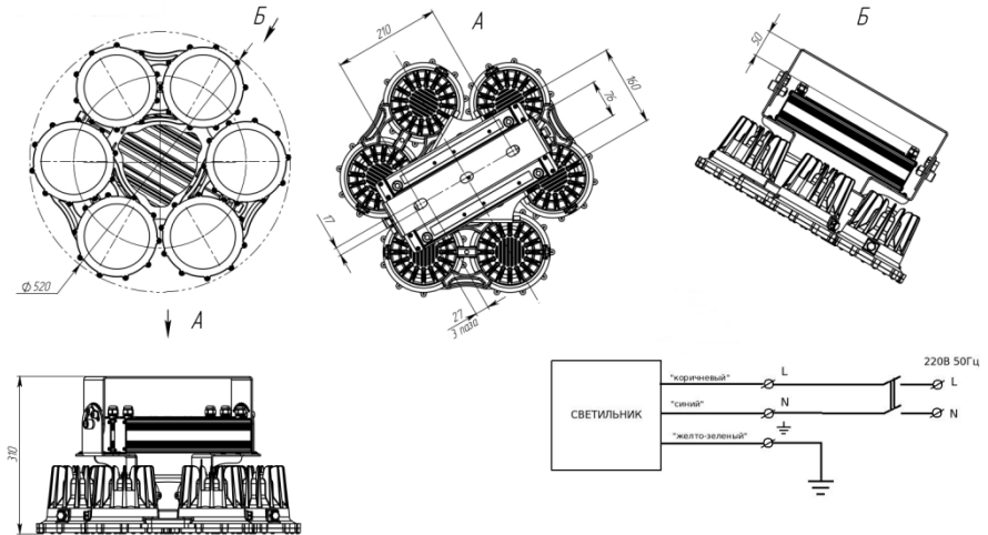
Рисунок 1. Габаритный чертеж.
